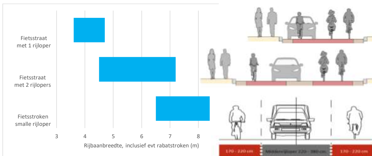
Figuur 5: Gewenste profielindeling voor een hoofd fietsroute op basis van gewenste rijbaanbreedte. Als de gewenste rijbaanbreedte groter is dan 6,5 meter, kan ook gekozen worden voor een profiel met fietsstroken en een smalle rijloper (zie de Fietsberaadnotitie “Aanbevelingen fiets- en kantstroken” uit 2015)
